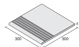
注文生産品 3. L-CD-R150K~R190K 300角階段平 2,400円/枚 平からの加工品
