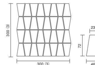
目地共寸法 300×300mm 4×8個/シート ※シート内の( ) 数字は目地幅を表しています。
